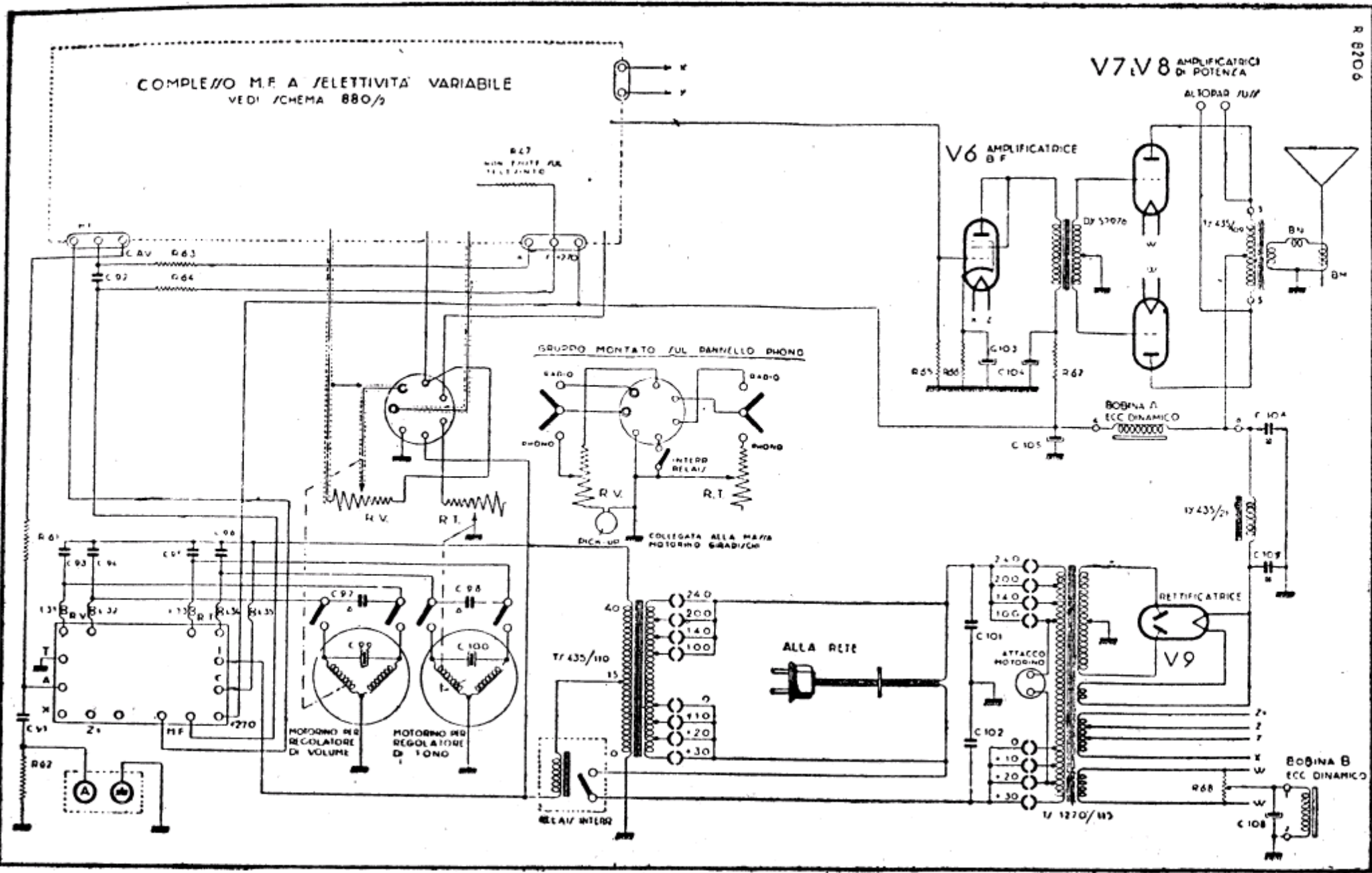
PHONOLA (S. A. FIMI) - Mod. « 910 ». - Particolari dell'amplificatore di bassa frequenza.
